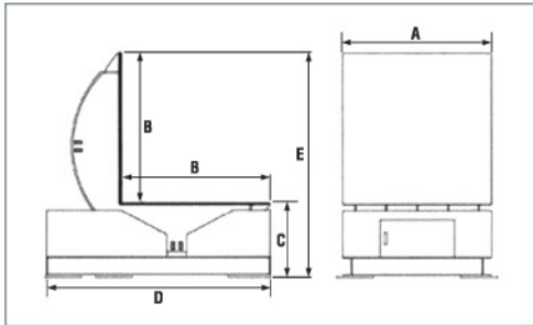
90도 반전기
