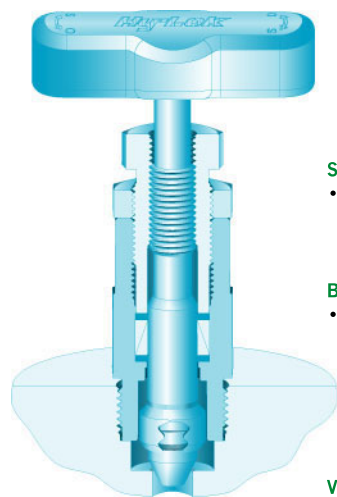
MBV Orifice 6.4
