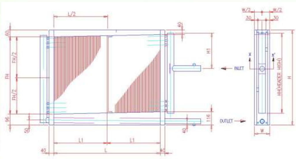
히팅코일 외형도
