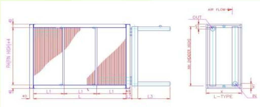
쿨링코일 외형도
