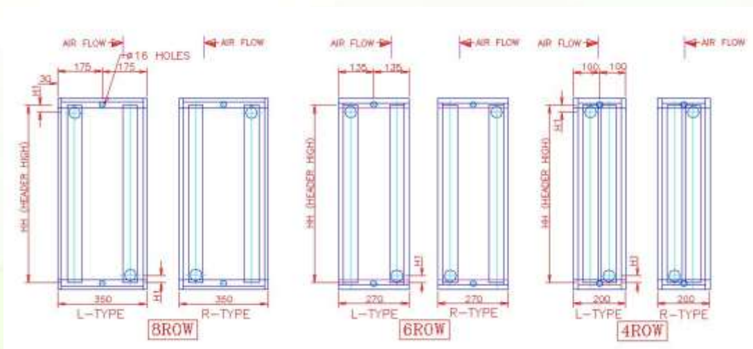
4,6,8ROW 코일 외형도
