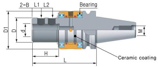
기본구성품(Basic Component)
