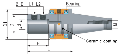
기본구성품(Basic Component)
