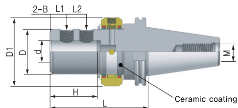
기본구성품(Basic Component)
