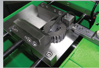
다이아몬드휠 기어절단
