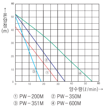
성능곡선도 (흡상높이 0.5m일 때)
