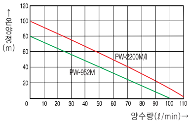
성능곡선도 (흡상높이 0.5m일 때)
