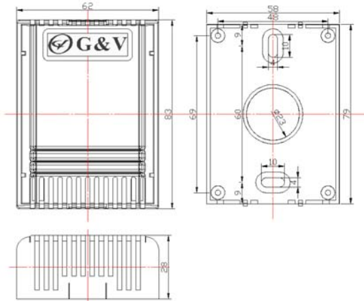
그림1 GHW-M20(R/T) 제품 치수
