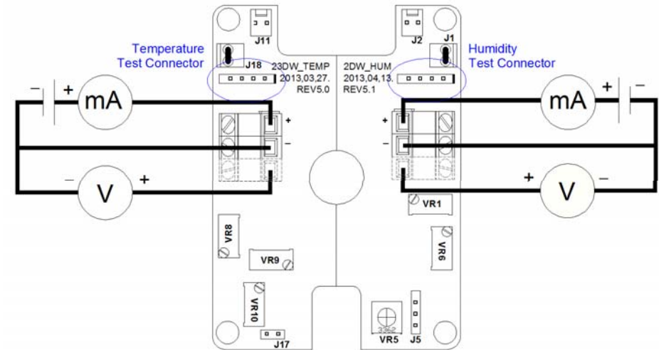
그림2 전기 결선도
