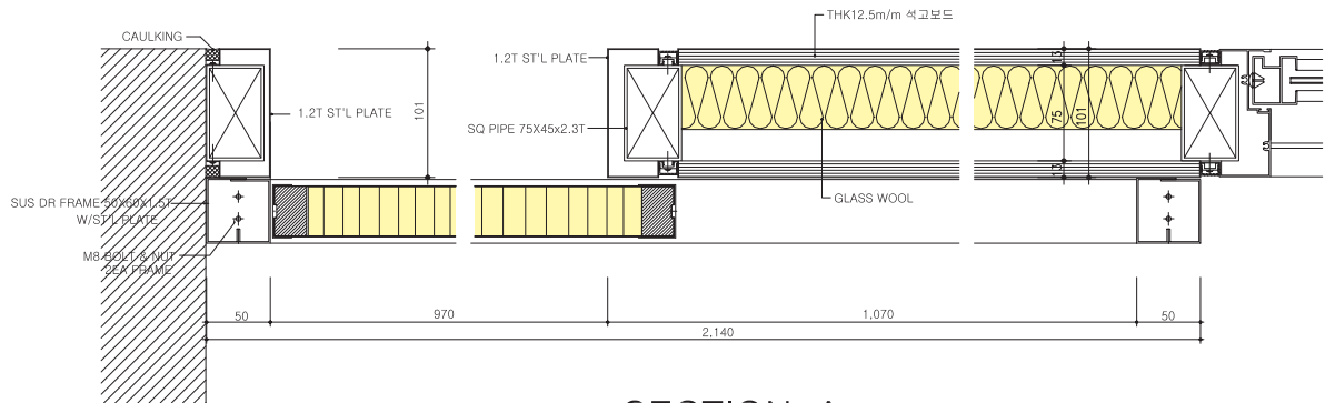
SECTION-A
