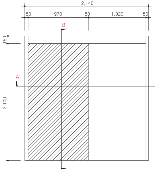
SLIDING DOOR ELEV.
